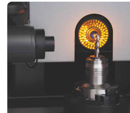
Измерение изготовленного инструмента
